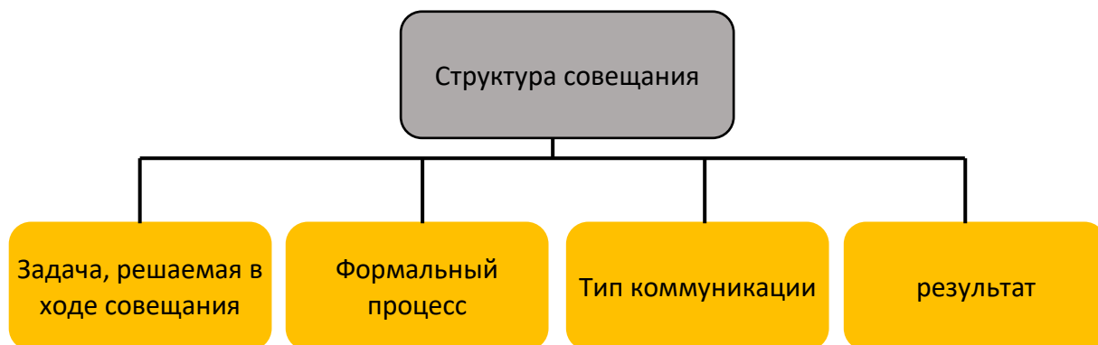
Рис. 3. Структура совещания
